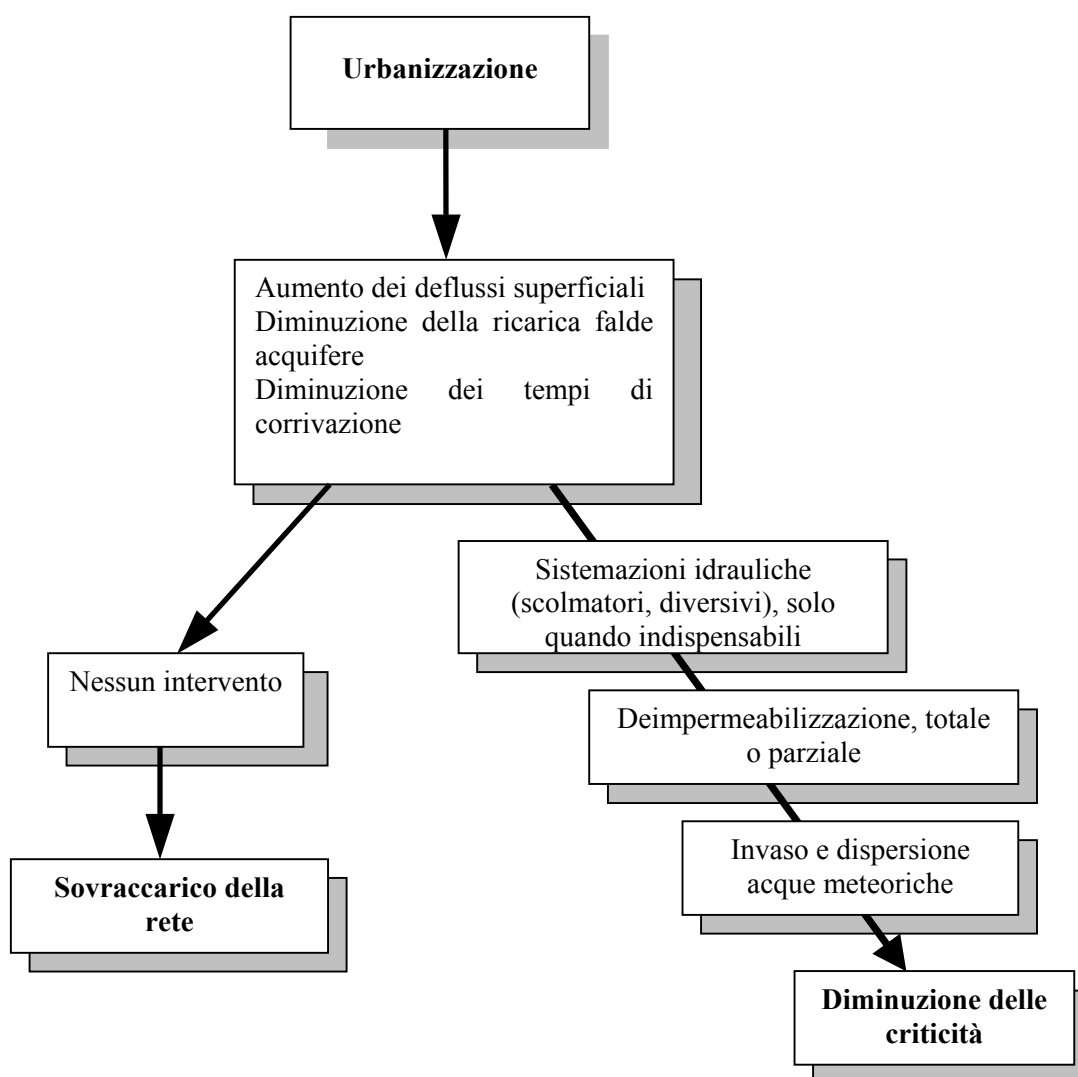
Figura 6-1 Indirizzi strategici per la difesa idraulica
