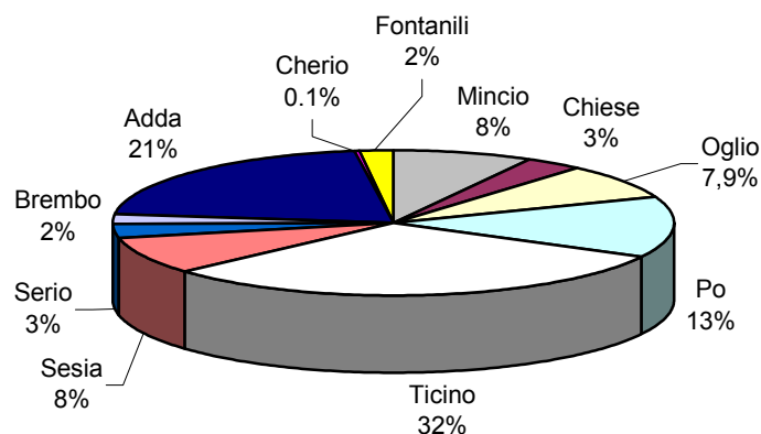
Figura 3-2 Ripartizione delle fonti irrigue in funzione delle portate derivate.
