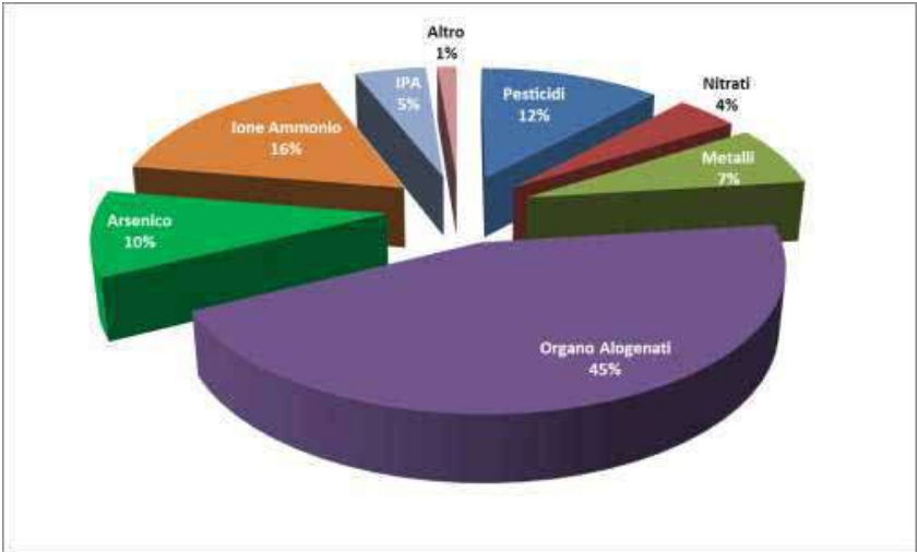
Figura 39 - Distribuzione percentuale dei superamenti di SQA o VS nel triennio 2012-2014 per le principali sostanze o gruppi di sostanze
