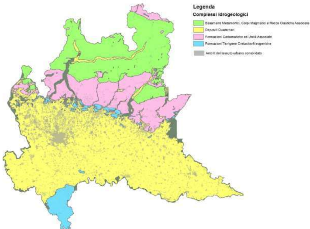
Figura 3 Corpi idrici sotterranei: individuazione dei complessi idrogeologici
