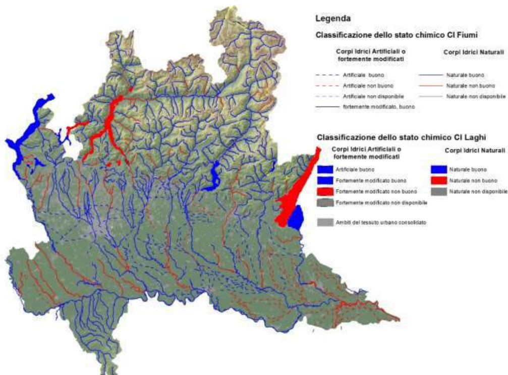
Figura 27 Corpi idrici superficiali: stato chimico
