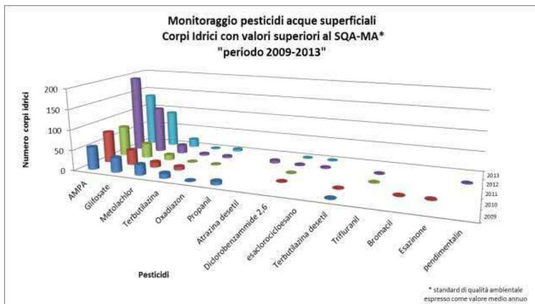
Figura 14 - Occorrenze di valori medi annui superiori agli SQA per le concentrazioni di pesticidi rilevate nelle acque superficiali nel periodo 2009-2013 tutte le sostanze
