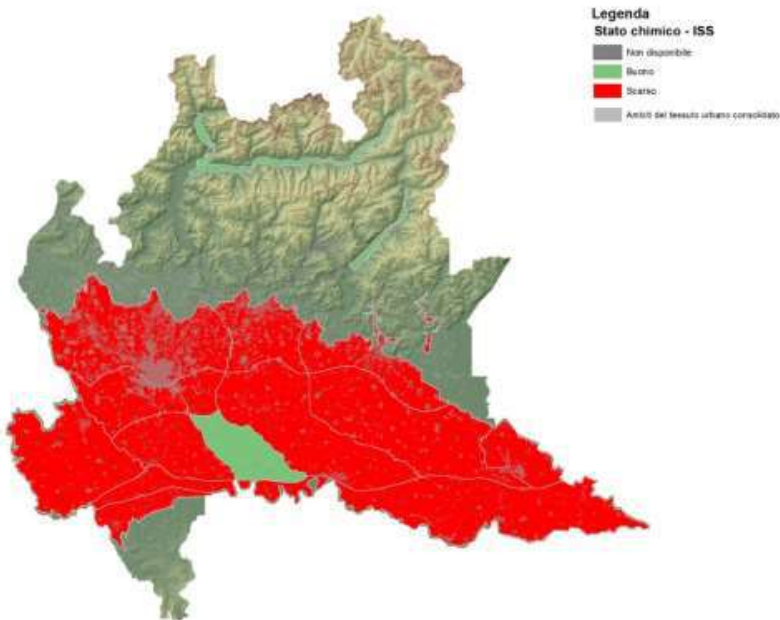
Figura 33 Corpi idrici sotterranei idrostruttura sotterranea superficiale: stato quantitativo
