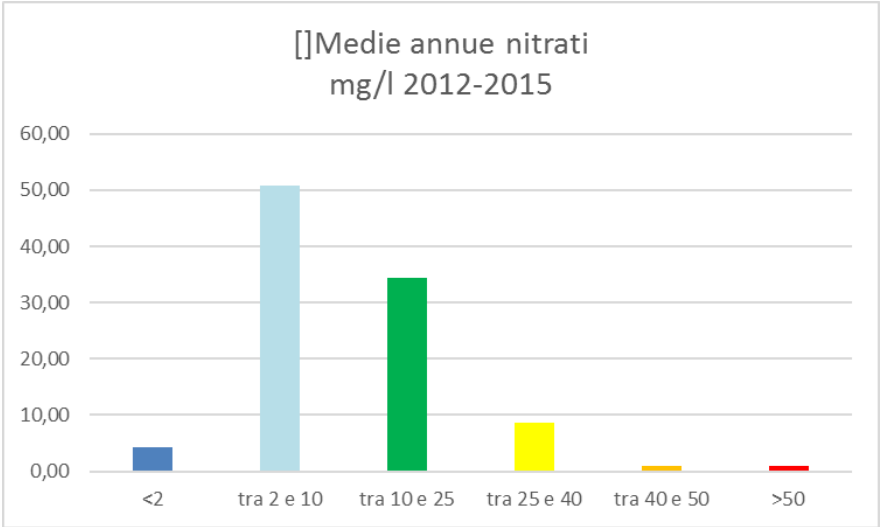
Figura 21 - Distribuzione (%) in classi delle concentrazioni medie annue di nitrati nel quadriennio di riferimento 2012-
