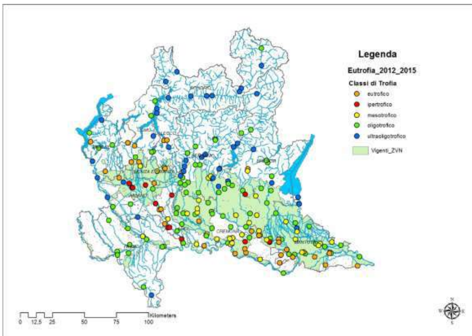
Figura 23 - Mappa delle distribuzioni in classi dello stato trofico nelle acque superficiali 2012-2015
