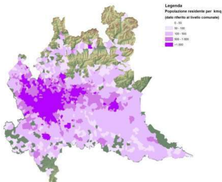
Figura 7 - Popolazione residente per Km 2
