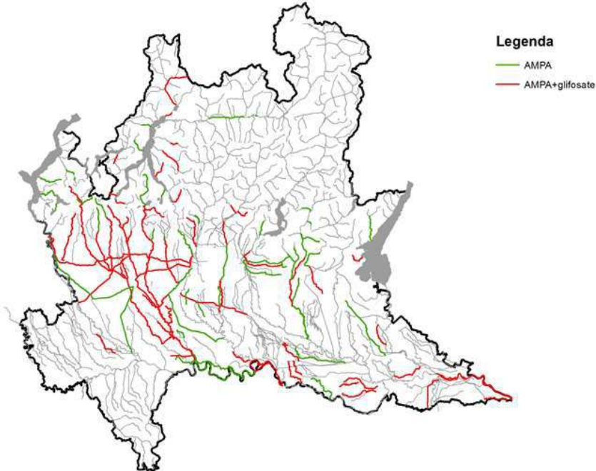
Figura 17 - Corpi idrici superficiali per i quali sono stati riscontrati superamenti degli SQA per la concentrazione media annua di AMPA e/o glifosate
