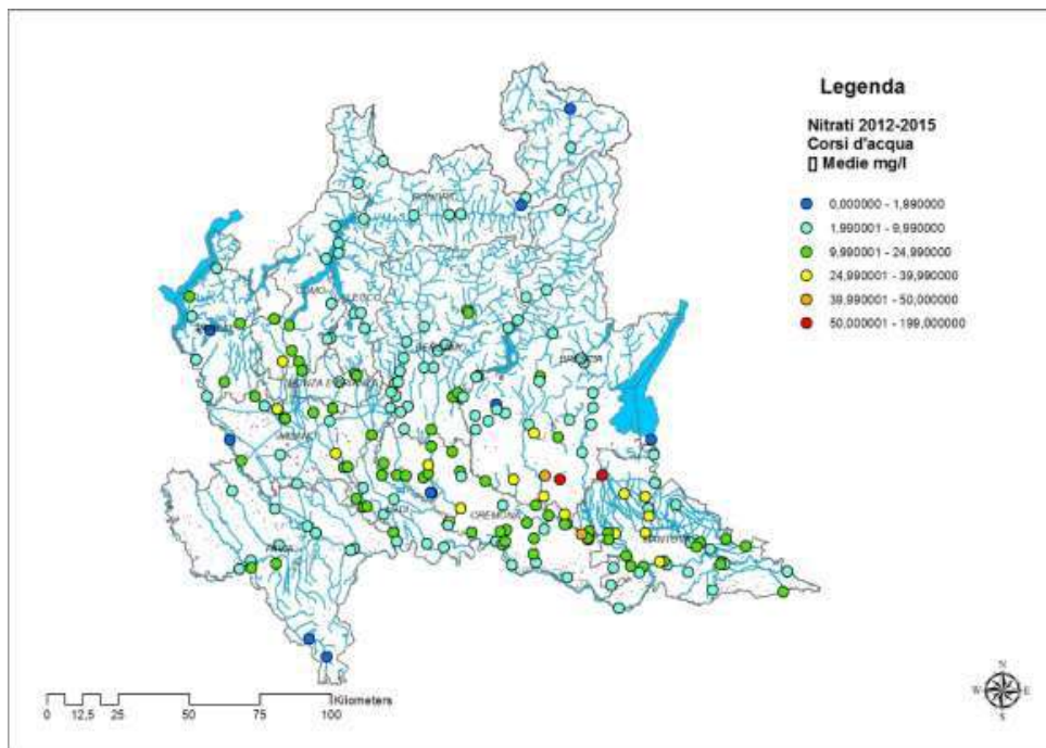
Figura 22 - Mappa delle distribuzioni in classi delle concentrazioni medie annue di nitrati (mg/l) nel quadriennio di riferimento 2012-
