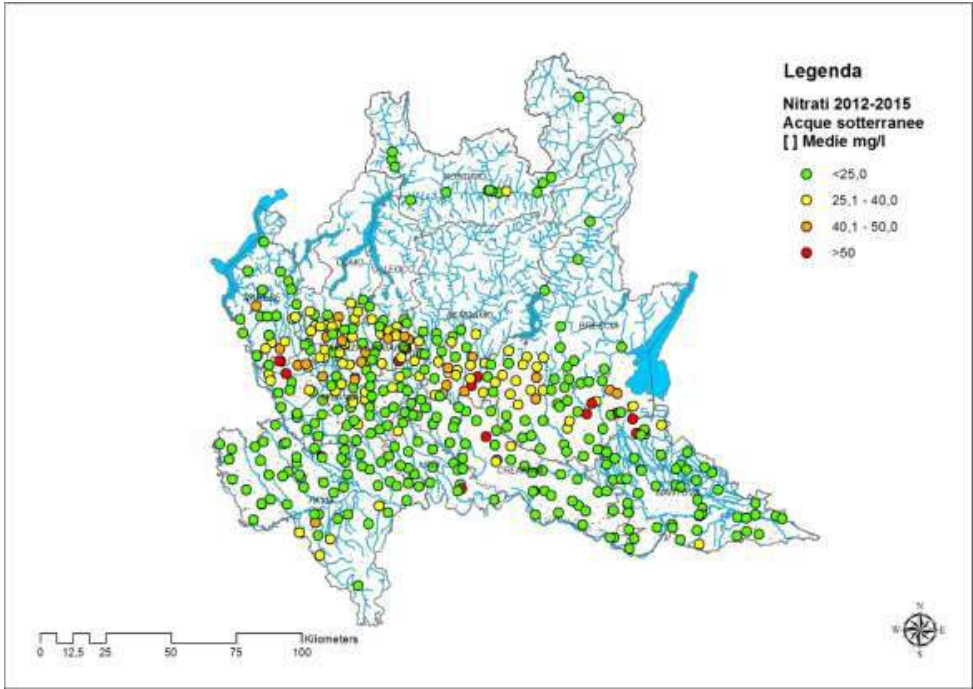
Figura 20 - Mappa delle distribuzioni in classi delle concentrazioni medie annue di nitrati (mg/l) nel quadriennio di riferimento 2012-2015 nelle acque sotterranee
