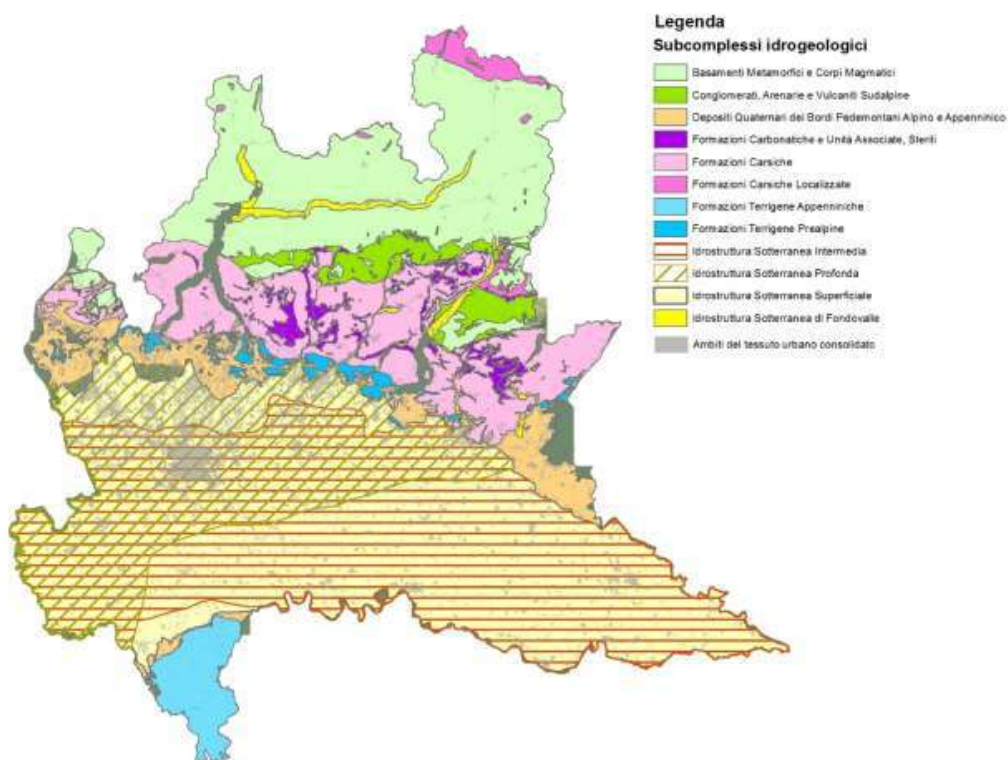
Figura 4 - Corpi idrici sotterranei: individuazione dei subcomplessi idrogeologici
