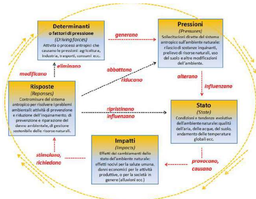
Figura 5 Il modello D.P.S.I.R.
