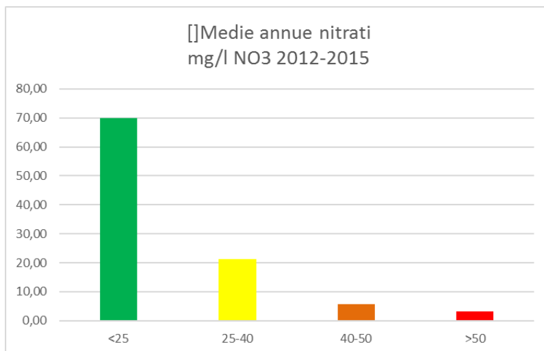
Figura 19 - Distribuzione (%) in classi delle concentrazioni medie annue di nitrati nel quadriennio di riferimento 2012-2015 nelle acque sotterranee
