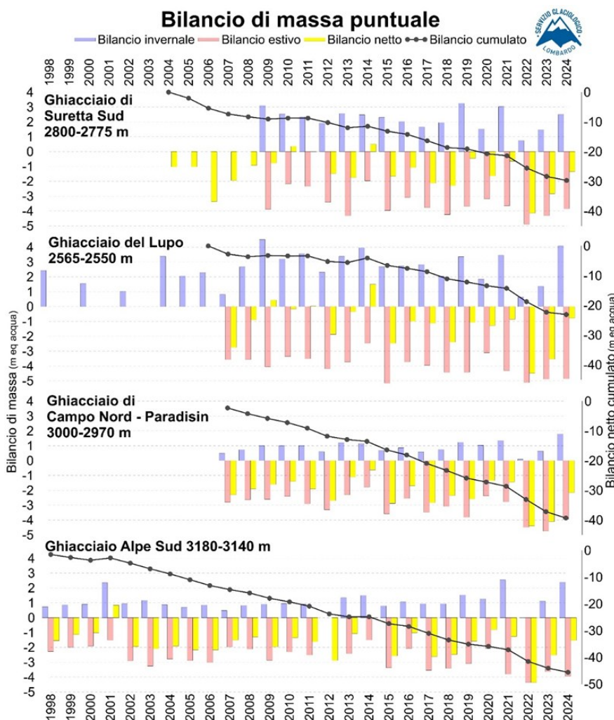
Figura 26 / Bilanci di massa puntuali su quattro ghiacciai campione della rete SGL.
